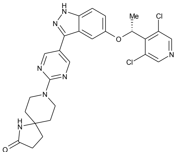
Приклад 48. 8-[5-[5-[(1R)-1-(3,5-дихлор-4-піридил)етоксі]-1H-індазол-3-іл]піримідин-2-іл]-1,8-діазаспіро[4,5]декан-2-он
