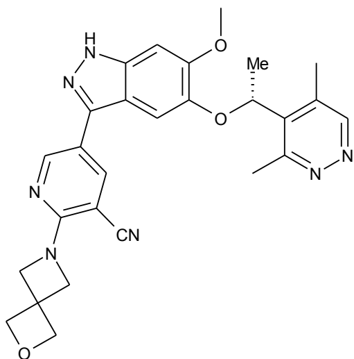
Приклад 218. (R)-5-(5-(1-(3,5-диметилпіридазин-4-іл)етокси)-6-метоксі-1H-індазол-3-іл)-2-(2-окса-6-азаспіро[3,3]гептан-6-іл)нікотинонітрил
