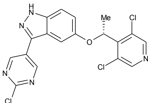
Приклад 59. 3-(2-Хлорпіримідин-5-іл)-5-[(1R)-1-(3,5-дихлор-4-піридил)етоксі]-1H-індазол
