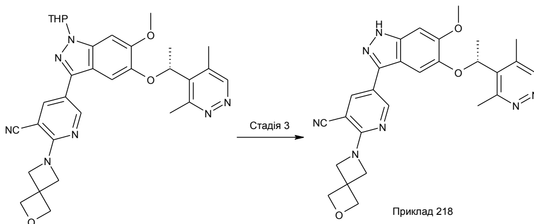
Приклад 218. (R)-5-(5-(1-(3,5-диметилпіридазин-4-іл)етокси)-6-метоксі-1H-індазол-3-іл)-2-(2-окса-6-азаспіро[3,3]гептан-6-іл)нікотинонітрил
