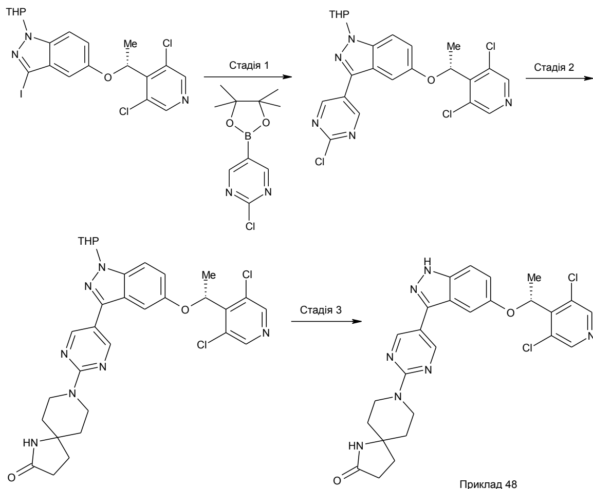
Приклад 48. 8-[5-[5-[(1R)-1-(3,5-дихлор-4-піридил)етоксі]-1H-індазол-3-іл]піримідин-2-іл]-1,8-діазаспіро[4,5]декан-2-он
