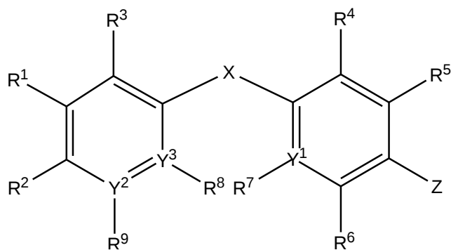
Формула (I)
