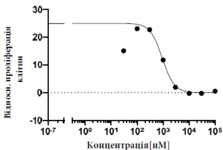
6-((4'-фтор-[1,1'-біфеніл]-4-іл)окси)-2-метилпіридин-3-амін
