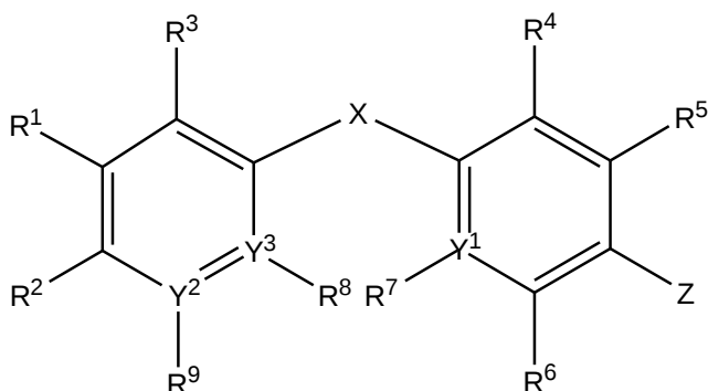
Формула (I)
