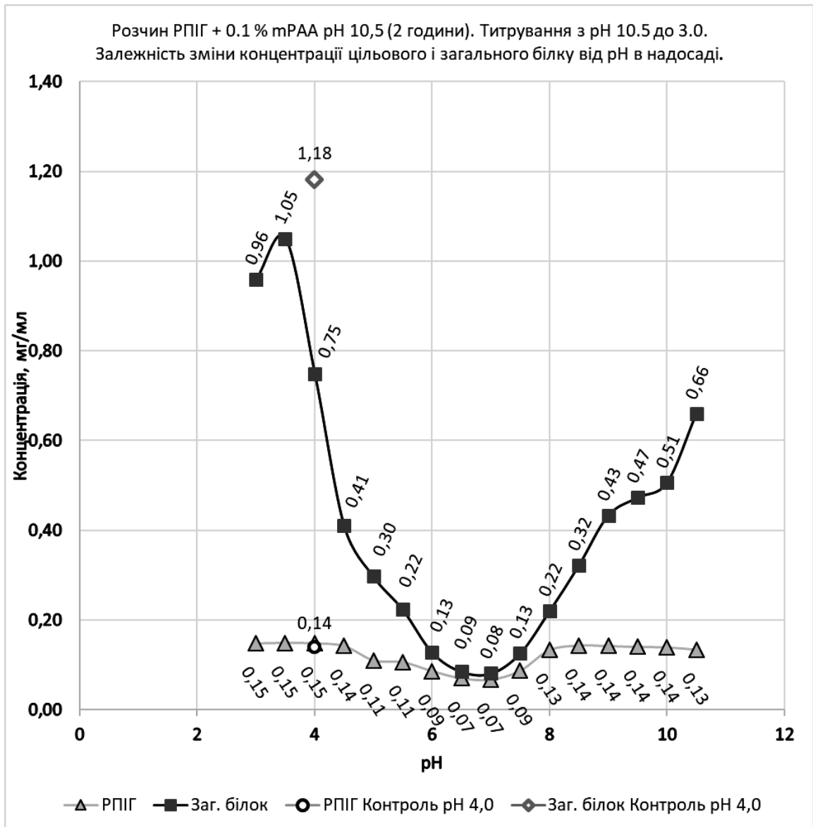
Фіг. 1. Графік «Залежність зміни концентрації цільового білку рефолдований попередник інсуліну гларгін і загального білку від значення pH в надосаді (фугаті)»
