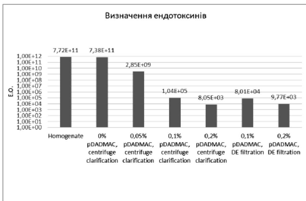
Фіг. 9. Графік «Визначення ендотоксинів». Визначення рівня ендотоксинів проводили з використанням комерційного набору ENDOLISA® (bioMérieux, Франція)
