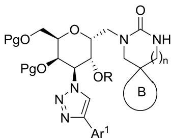
Структура 1с (циклічна сечовина)
