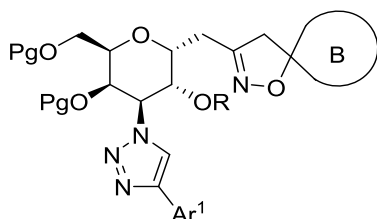
Структура 1a (ізоксазолін)
