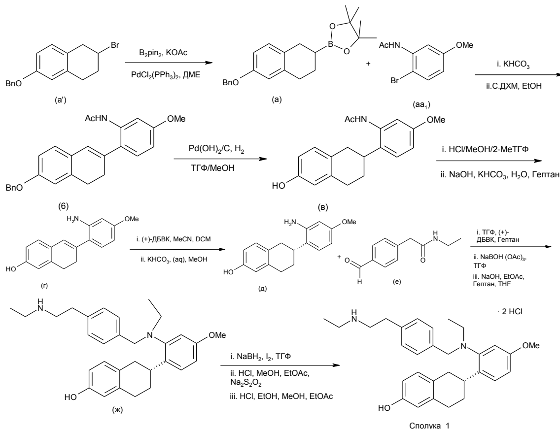
Схема 1 - Одержання сполуки 1 2\text{HCl}
