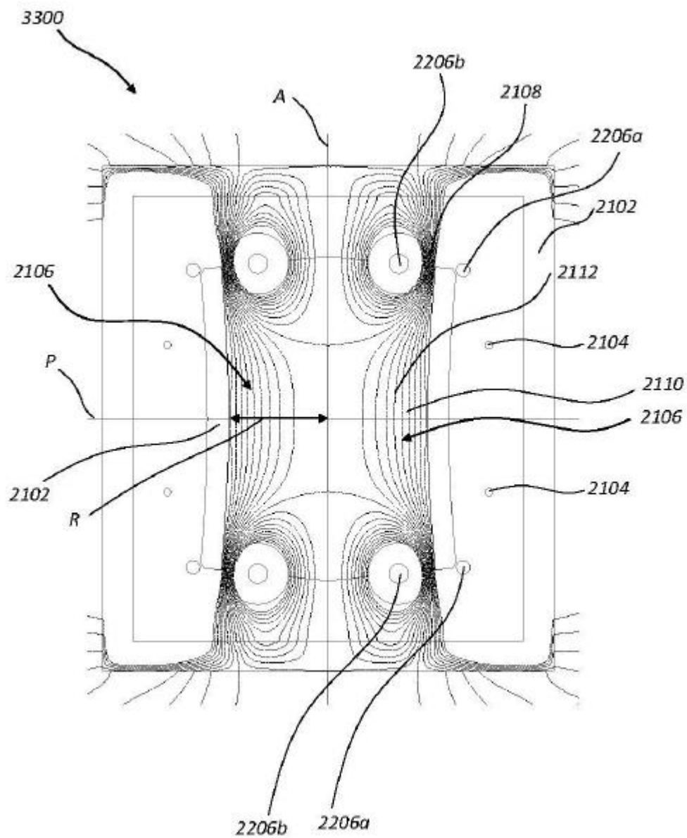
Φir. 23A
