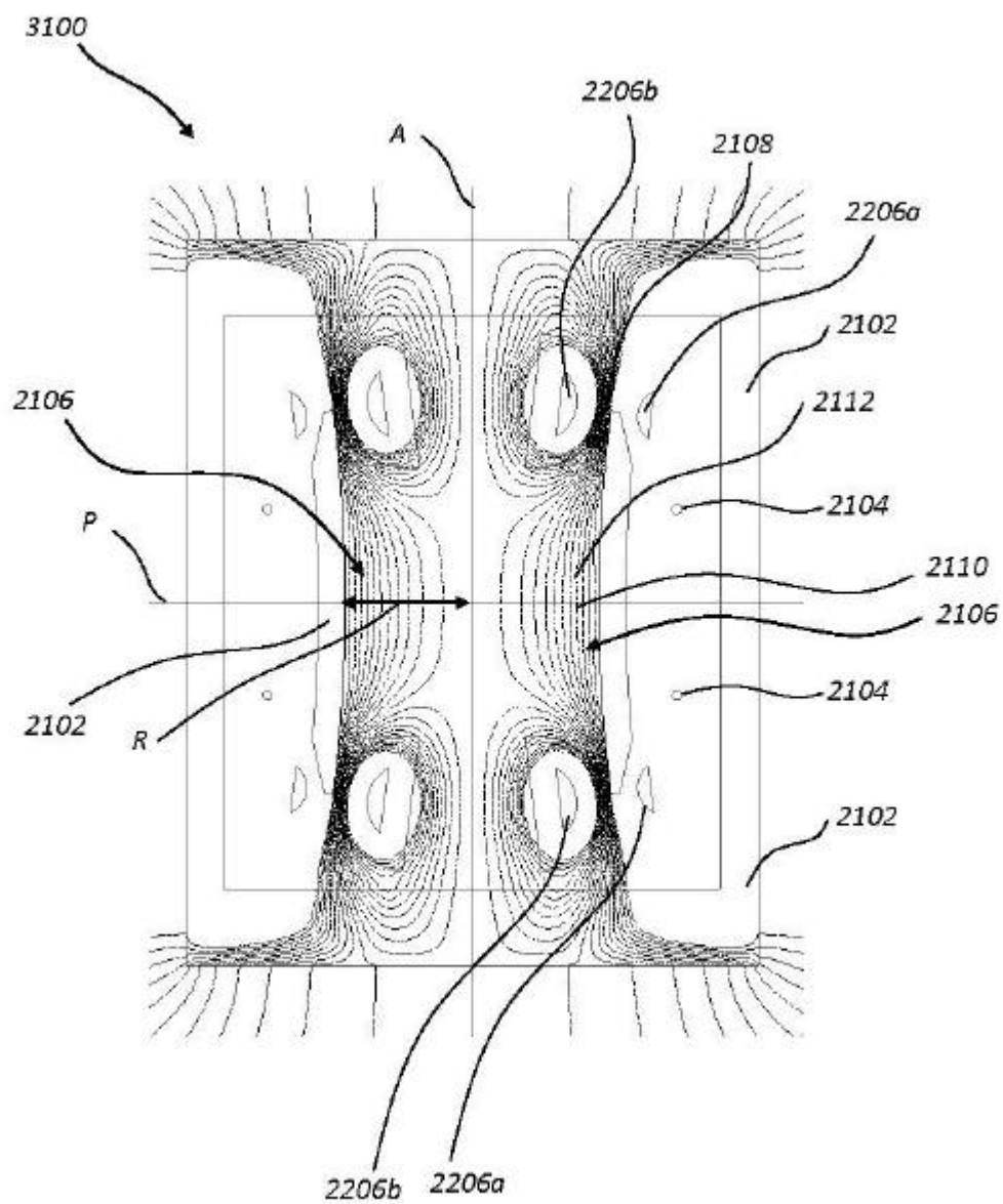
Fig. 21A
