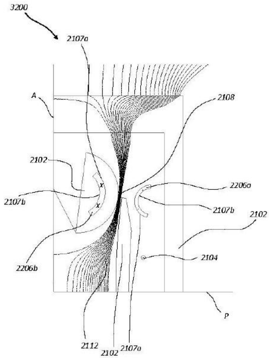
Φir. 22B
