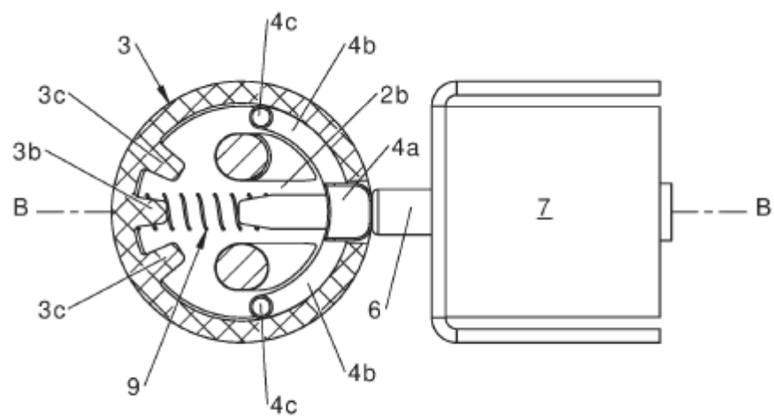
Фиг. 9
