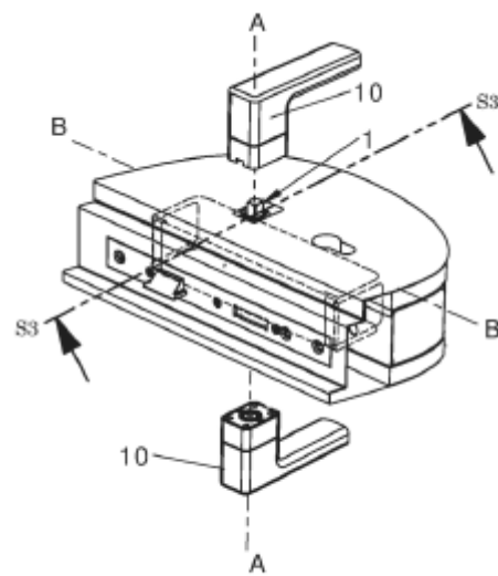
Фиг. 13
