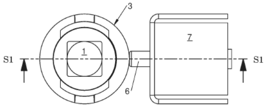
Фиг. 7
