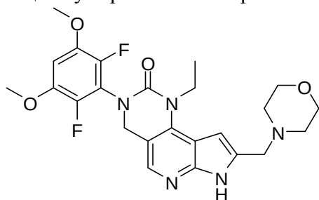
Сполука 1.
