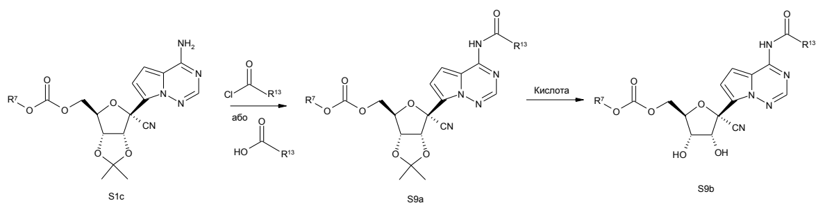
Схема 9
