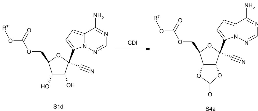
Схема 4
