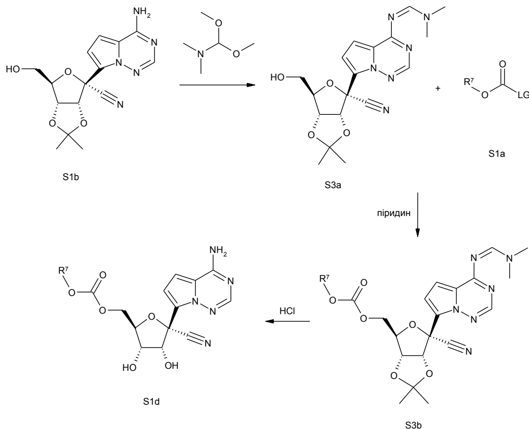
Схема 3
