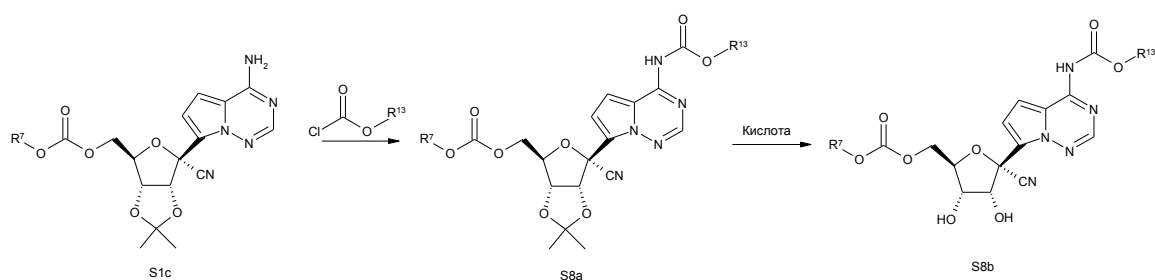
Схема 8
