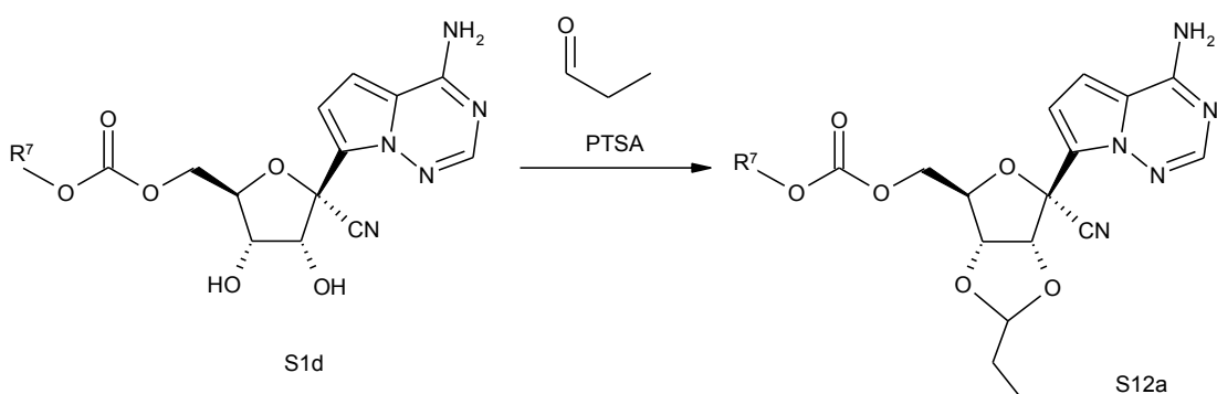
Схема 12
