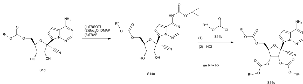
Схема 14
